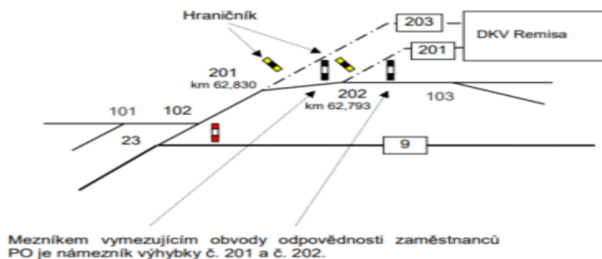
Plánek vlečky na styku drah
